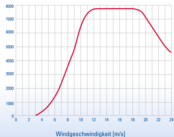
Leistung [kW]
